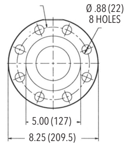
316SS 3" Class 300 R.F.
